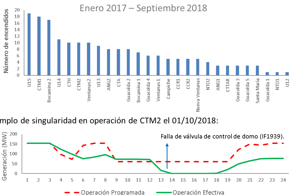
Figura 29: Número de encendidos o reconexiones de unidades a carbón después de no estar inyectando energía al sistema durante un periodo menor o igual a 8 horas. Fuente: Elaboración Propia
